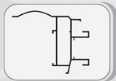
Série 20225 R Dormant avec couvre joint
